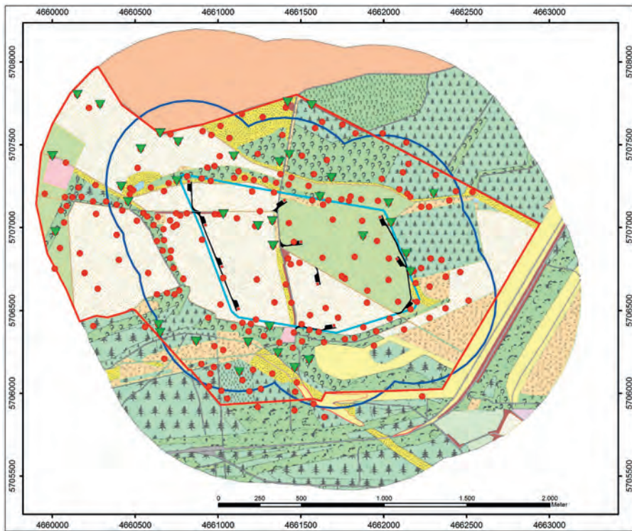
Abb. 6: Übersicht zur Brutvogelkartierung 2004. Darstellung aller 232 Reviermittelpunkte (400-ha-Fläche; rote Linie) mit wertgebenden Arten (grüne Dreiecke) in Bezug zum Windpark (hellblau) und dem 500-m-Umkreis (dunkelblau).
